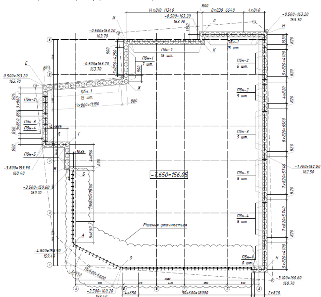
Рис.1 Схема конструкцій огороження котловану
