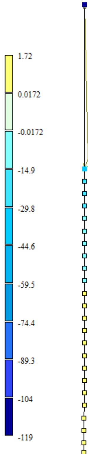
Рис.5. Переміщення палі після статичного розрахунку.
